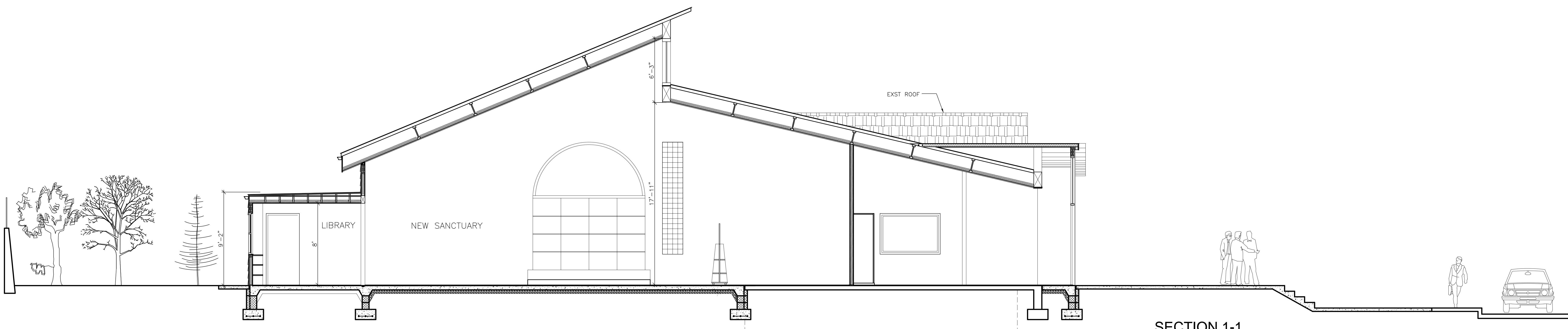
SECTION B-B SCALE: 1/4" = 1'-0"
